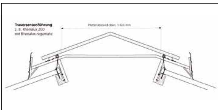
Traversenauführung z.B. Rhenalux 200 mit Rhenalux-regumatic
