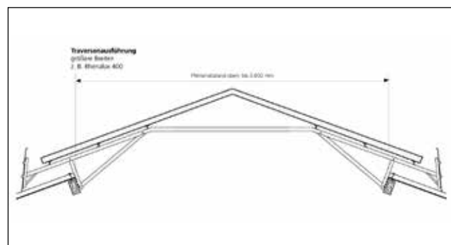
Traversenauführung größere Breiten z.B. Rhenalux 400
