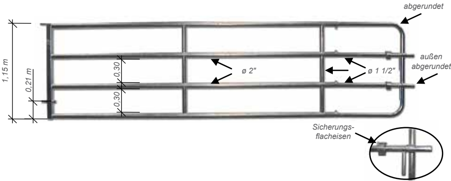
Bei Teleskoptüren < 1,65 m muss das Einsteckteil bauseits eingekürzt werden!
