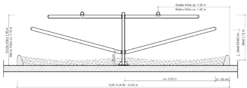
Doppelliegebox (Tiefbox)
