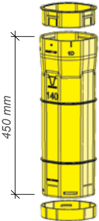
TR4140 Einbauhülse Ø 140 mm mit Dichting und Boden.
